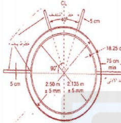
شكل دائري رمي القرص ورمي المطرقة المتماثلين
