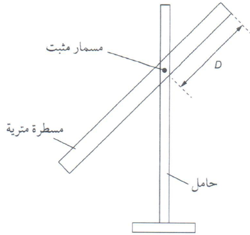
الشكل ٧-١١: نموذج تجريبي لمسطرة مترية تم تعليقها بواسطة مسمار رفيع يمر من خلال ثقب.
