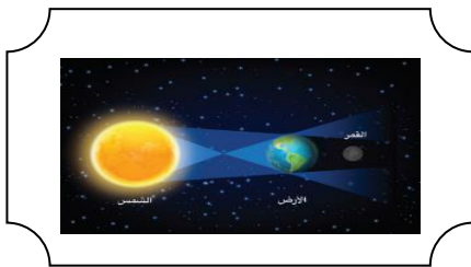
الخسوف
