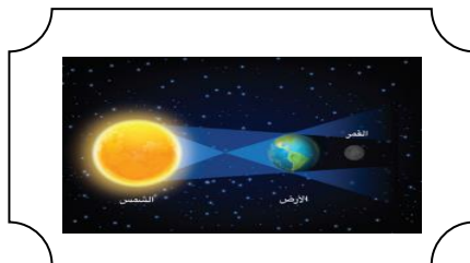
الخسوف
