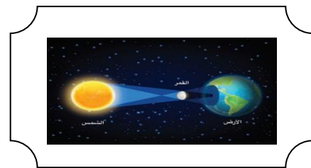
الكسوف
