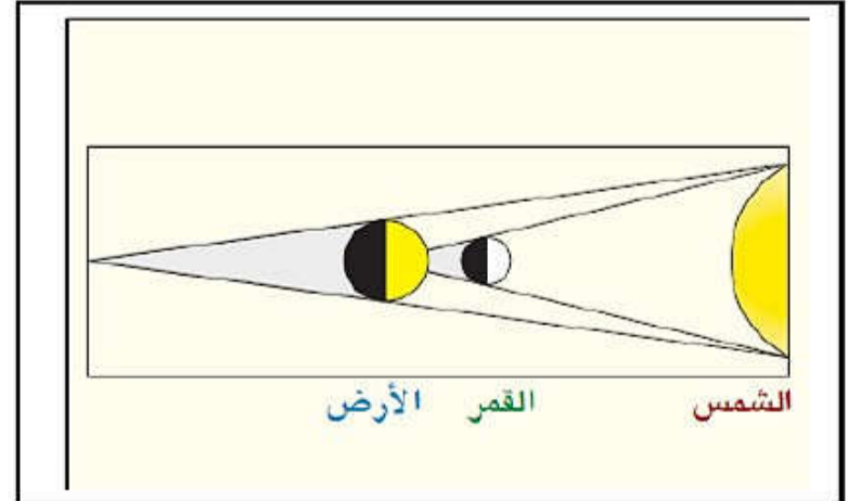
ظاهرة الكسوف
